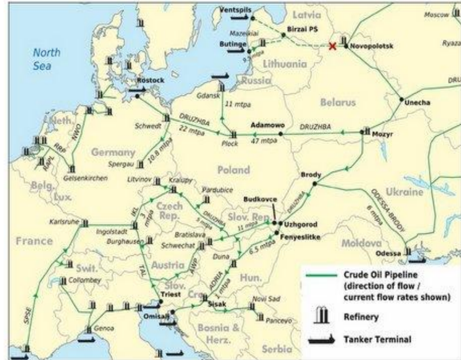
Sieť ropovodov a hlavných rafinérií v Strednej a Východnej Európe Aktuálne využitie kapacít ropovodov v mil. ton ropy ročne
